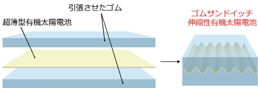
図 4 ゴムサンドイッチ構造による高い耐水性を持つ伸縮性有機太陽電池
